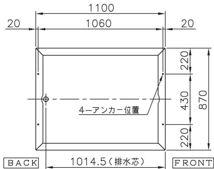
15WS架台伏せ図
