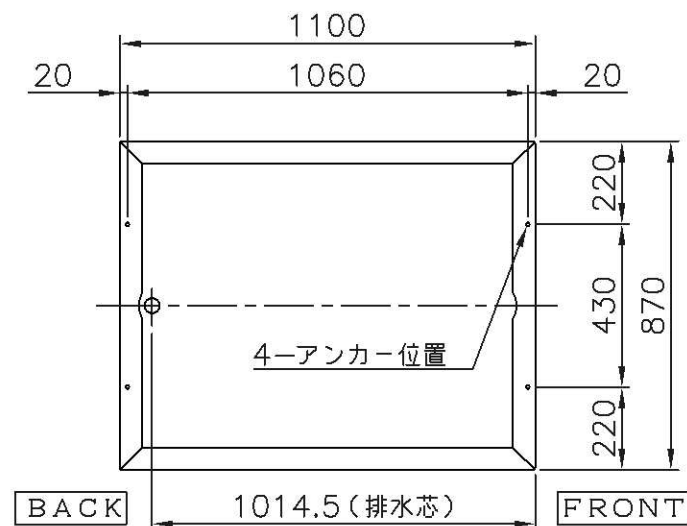
15WS架台伏せ図
