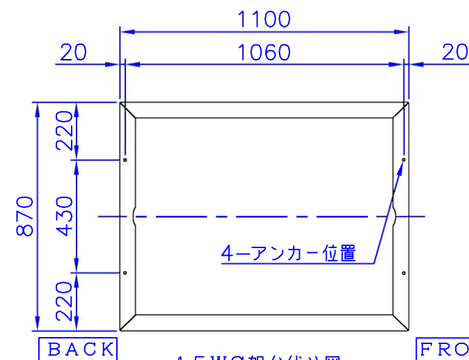
15WS架台伏せ図
