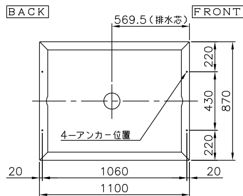
15WS架台伏せ図
