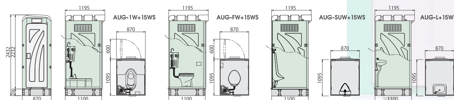
壁排水
